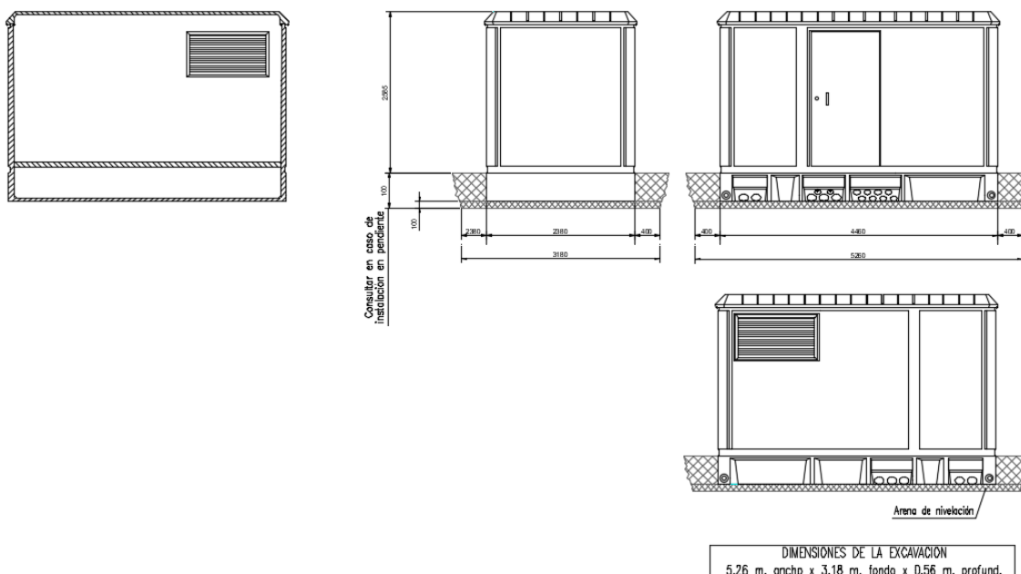
Ilustración 3. Centro de Entrega PFV La Bardina 2 y su ampliación 15 kV
